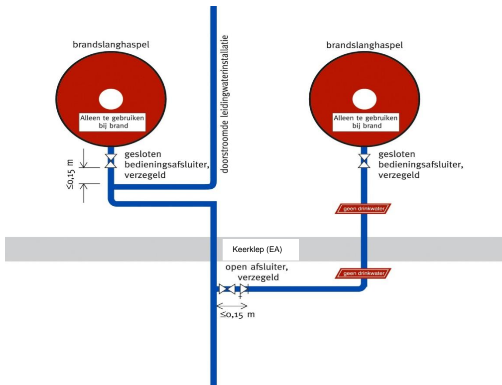
Figuur 2 Principeschets geen separate bluswaterleiding
