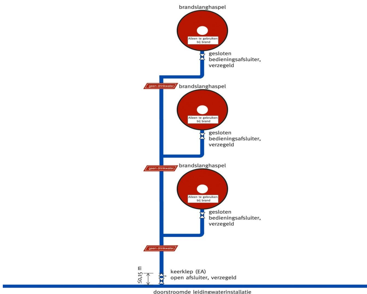
Figuur 1 Principeschets separate bluswaterleiding
